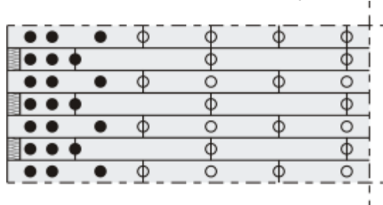
14 hmoždinek /m 2 na nároží objektu
