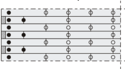
12 hmoždinek/m 2 na nároží objektu
