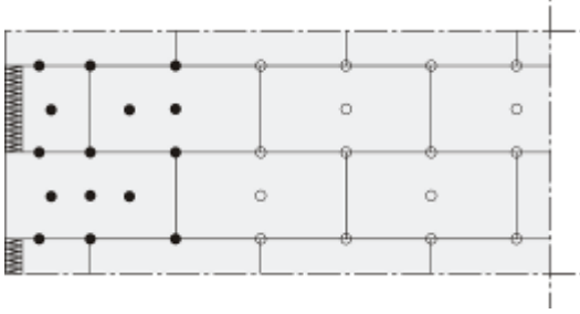
10 hmoždinek/m 2 na nároží objektu
